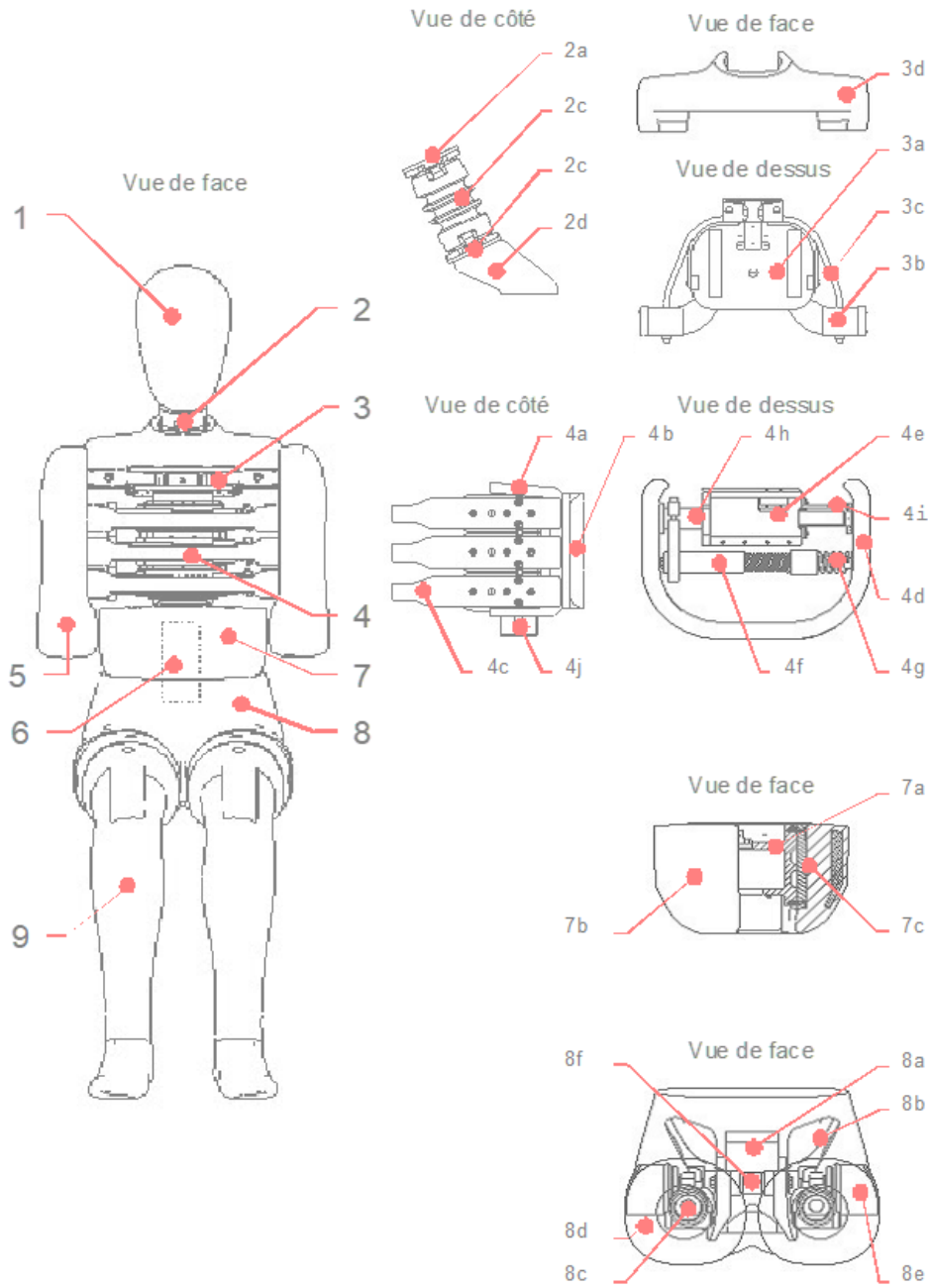
Figure 1 Structure du mannequin pour essais de choc latéral
