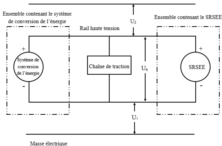
Figure 1 Mesure de U_b , U_1 et U_2
