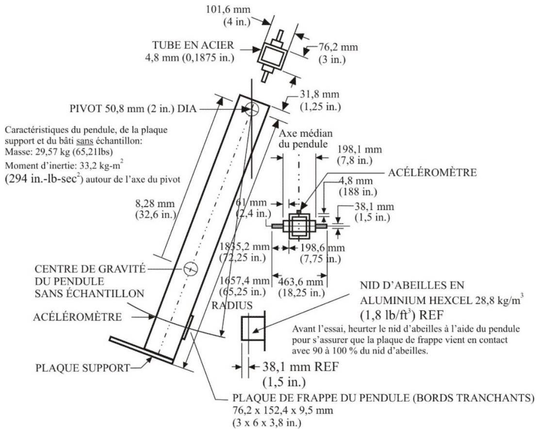
Figure 5 Caractéristiques du pendule cervical conformément au Règlement fédéral n° 49 des États-Unis, chapitre V, partie 572.33
