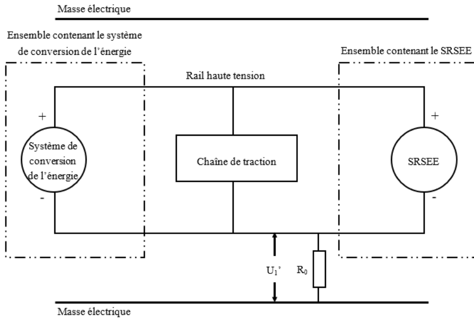
Figure 5 Mesure de U_1'
