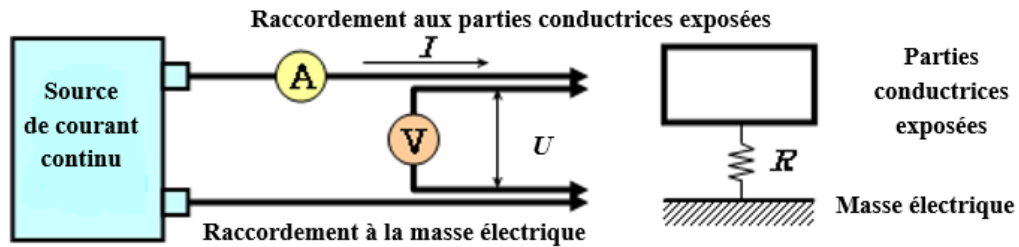
Figure 4 Exemple de méthode d'essai utilisant une source de courant continu
