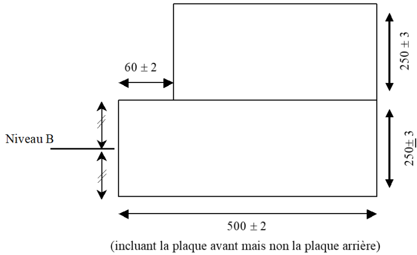
Figure 3 Orientation de la structure alvéolaire en aluminium
