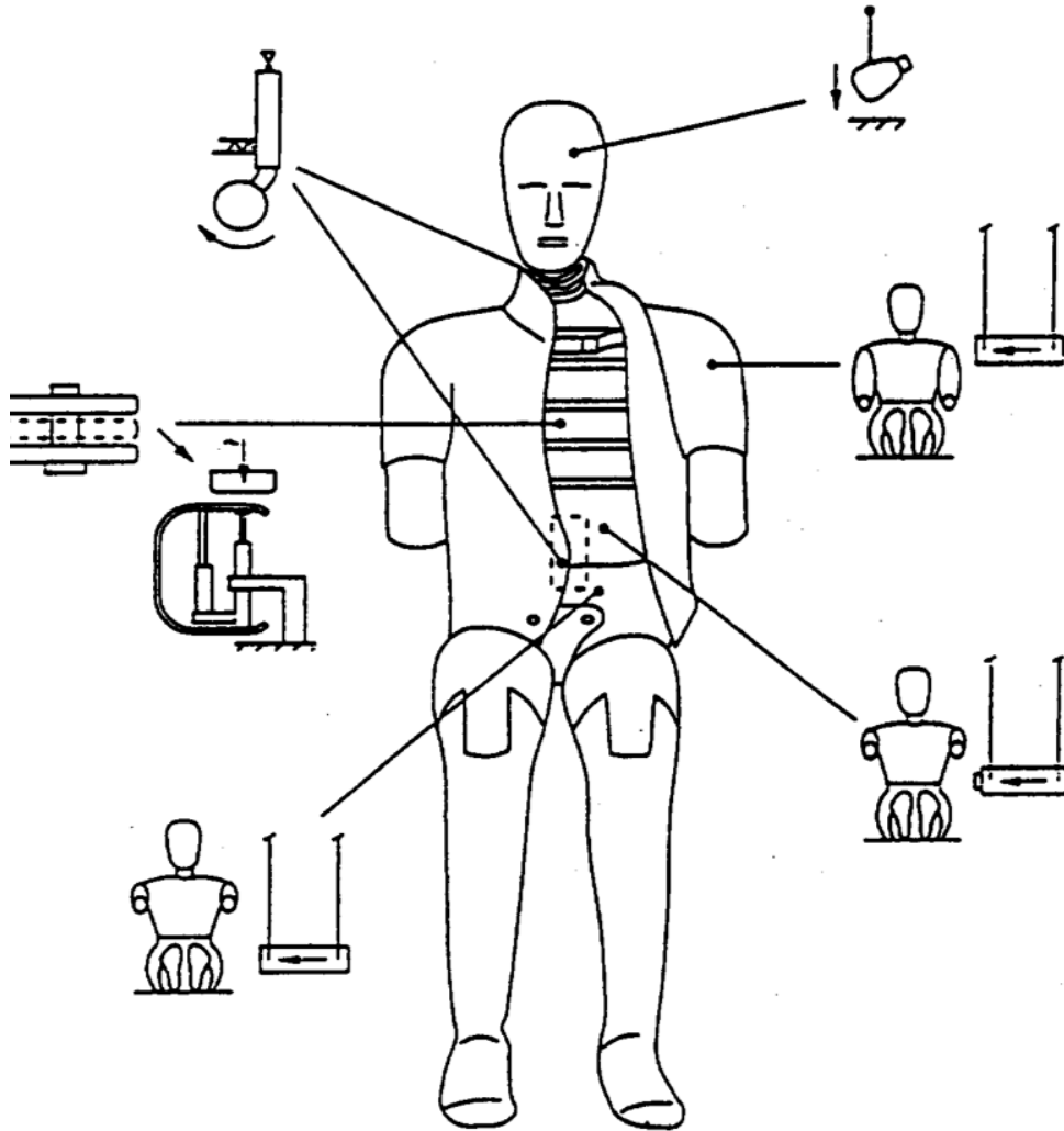
Vue d'ensemble du montage pour l'essai d'homologation du mannequin de choc latéral
