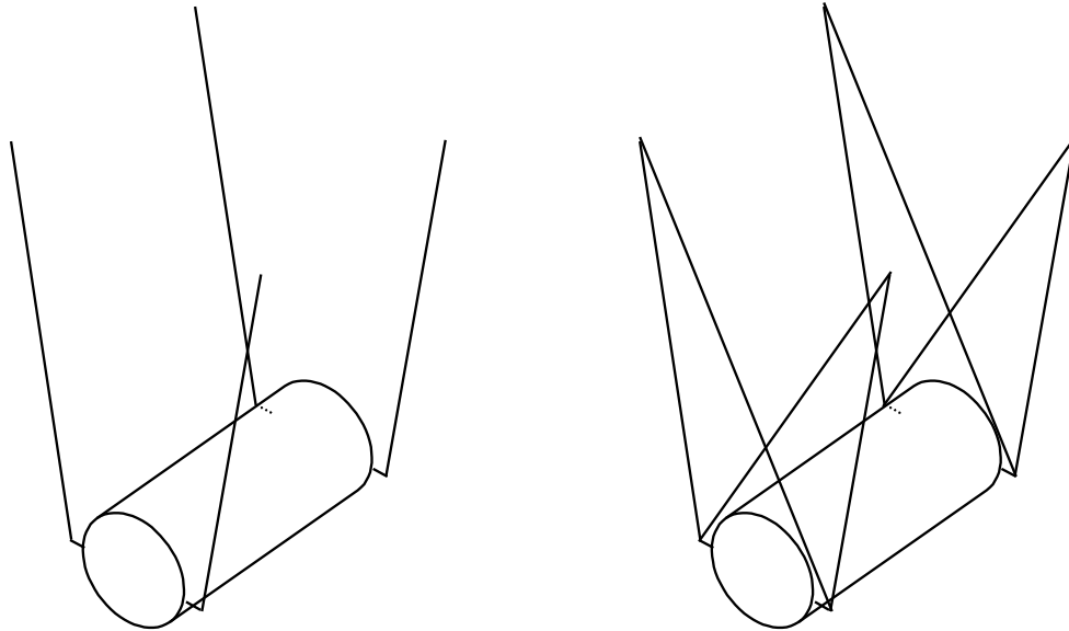
Figure 5 Caractéristiques du pendule cervical conformément au Règlement fédéral n° 49 des États-Unis, chapitre V, partie 572.33
