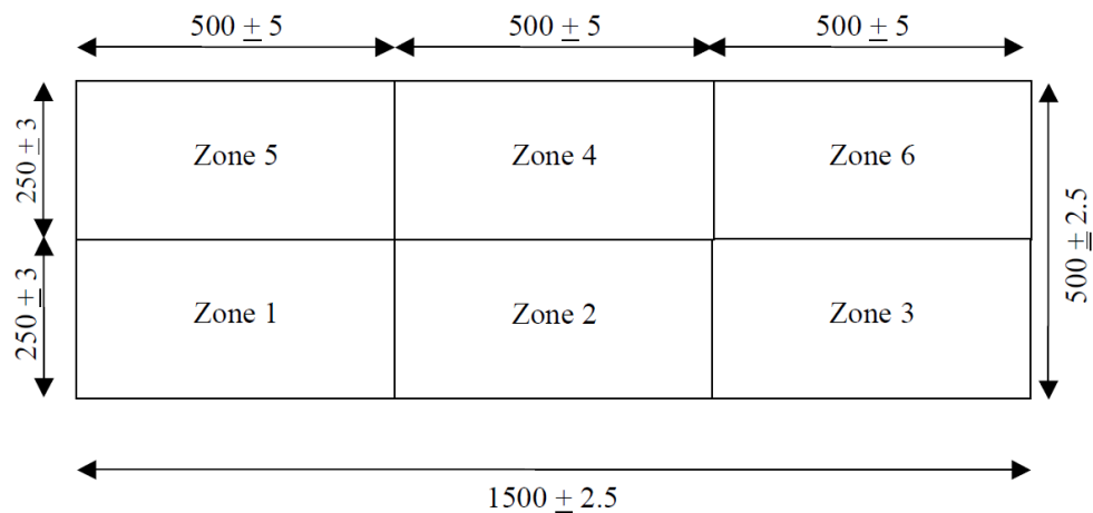
Figure 1 Conception de l'élément de frappe 2
